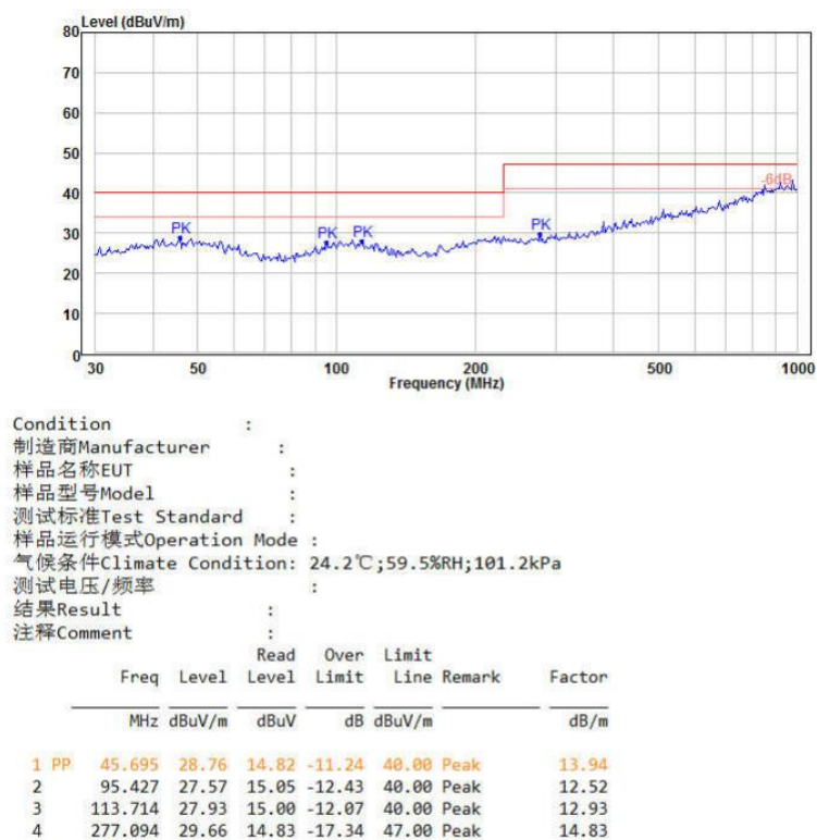
图 7-6 辐射测试水平方向
