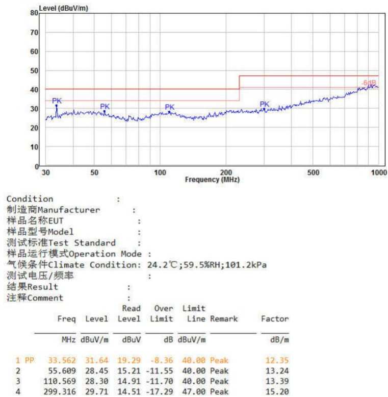
图 7-7 辐射测试垂直方向
